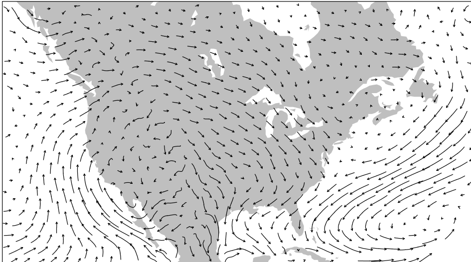
Mercator - NARR
